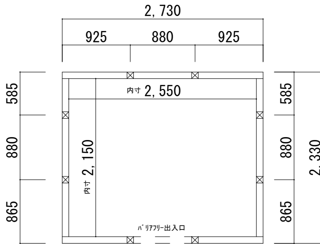
土台伏図
