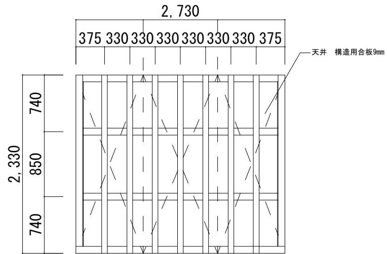
屋根伏図
