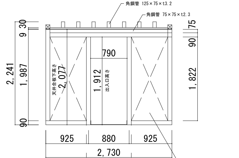
正面図
