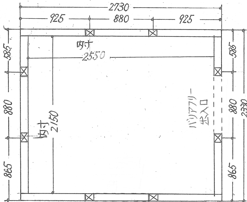
土台伏図
