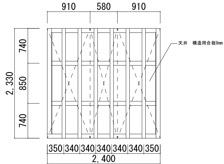
屋根伏図
