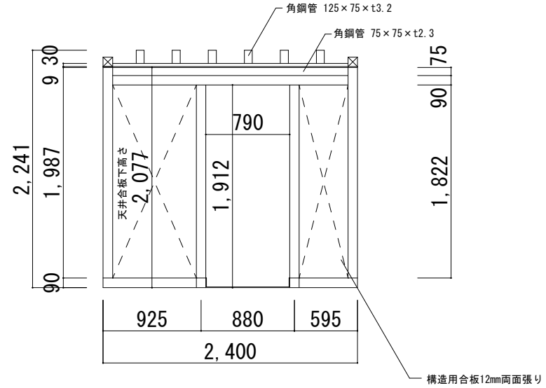
正面図
